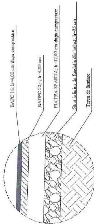
Detaliu A - A SCARA 1:25
